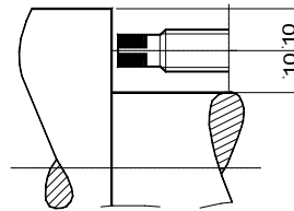
Abstand zur Wellenschulter Sensor parallel zu elektrisch leitfähigem Material Distance to shaft shoulder Sensor parallel to electrically conducting material Distance à l'épaule d'arbre Capteur monté en parallèle à un matériel conducteur
