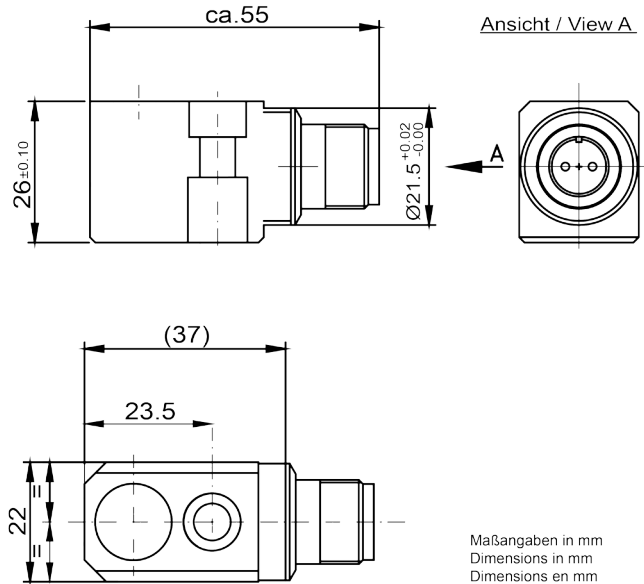
Abb. 1: Beschleunigungs-Sensor Fig. 1: Acceleration Sensor Fig. 1: Accéléromètre
