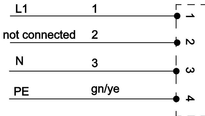
Abb.2: Anschluss
